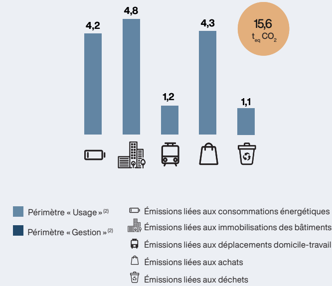
BILAN CARBONE DU SIÈGE ALLOUÉ PAR PRINCIPAUX POSTES D'ÉMISSIONS (3)
