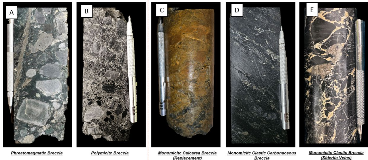
Figure 6-7: Different Types of Breccias in San Gabriel. A) Phreatomagmatic breccia. B) Polymictic breccia. C) Monomictic calcarea breccia. D) Monomictic clastic breccia. E) Monomictic clastic breccia.
